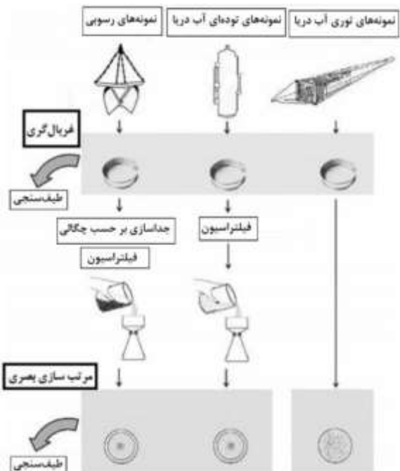
شکل ۳- روش‌های مختلف نمونه‌برداری از میکروپلاستیکها در محیط‌های مختلف و مراحل پردازش نمونه‌ها (Ruz et al. 2012) Fig. 3 Different methods of sampling microplastics in different environments and process stages of samples (Ruz et al. 2012)
