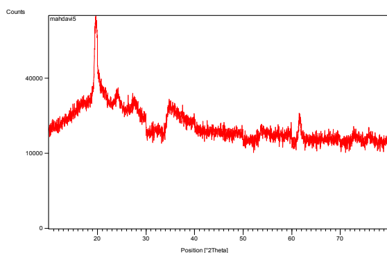
شکل ۱- الگوی XRD نانورس مونت موریلونایت (قبل از جذب سولفات)
