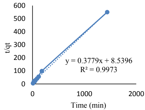
شکل ۴ - مدل سینتیکی شبه‌مرتبه دوم جذب سولفات Fig. 4 Pseudo-second-order kinetic model of sulfate adsorption
